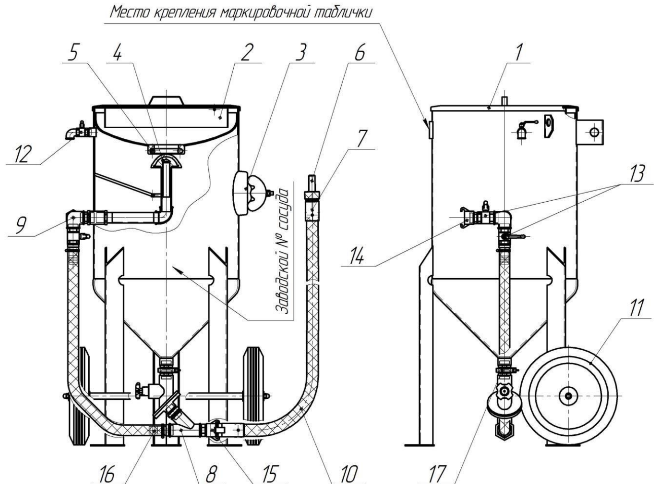
Установка «GN» ® без КПДУ
